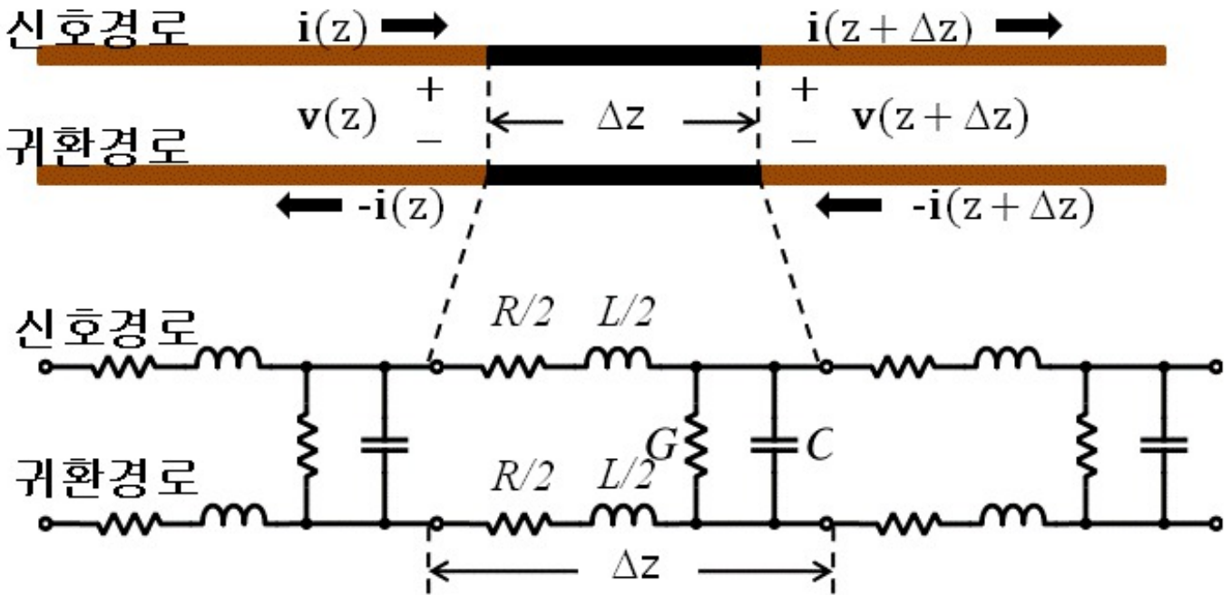
(a) 전송선 \Delta z 부분에 대한 등가회로
