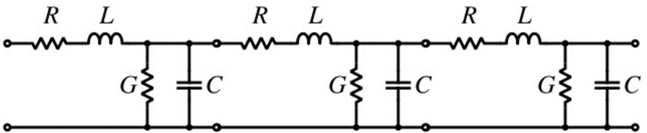
(b) 귀환경로의 R 과 L 을 합친 등가회로
